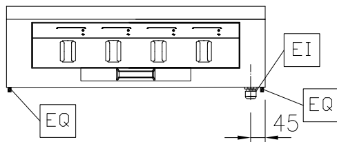
Front aanzicht
