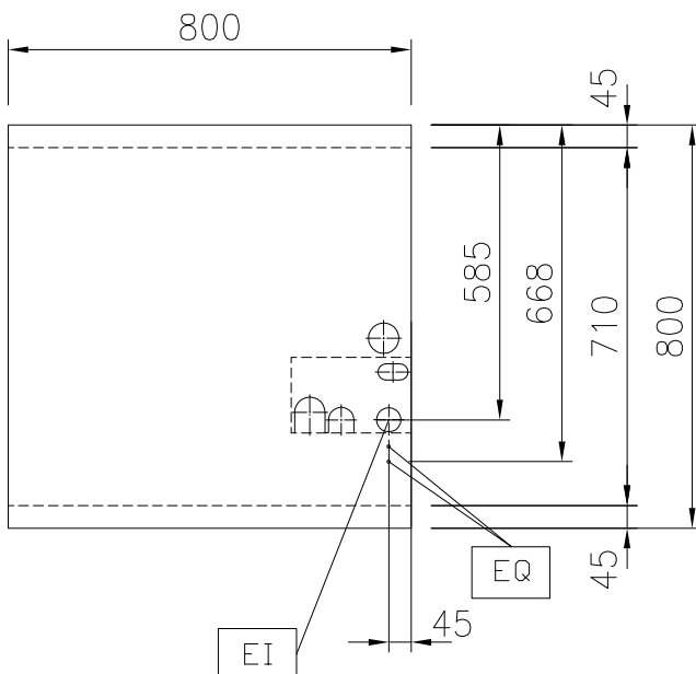
Boven aanzicht
